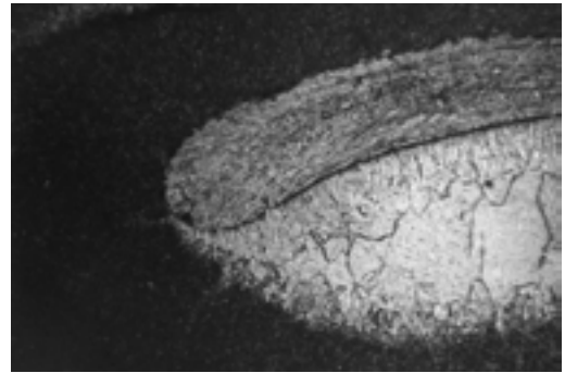
Abb. 5: Zement-Calcitfüllung in ehemaligen Hohlraum unter einer Muschelschale. Die feinkörnige Kalkmasse der Lumachelle erscheint im Bilde schwarz. Dünnschliff unter dem Pol.-Mikroskop. Bildausschnitt: 2,4 x 1,7 mm
