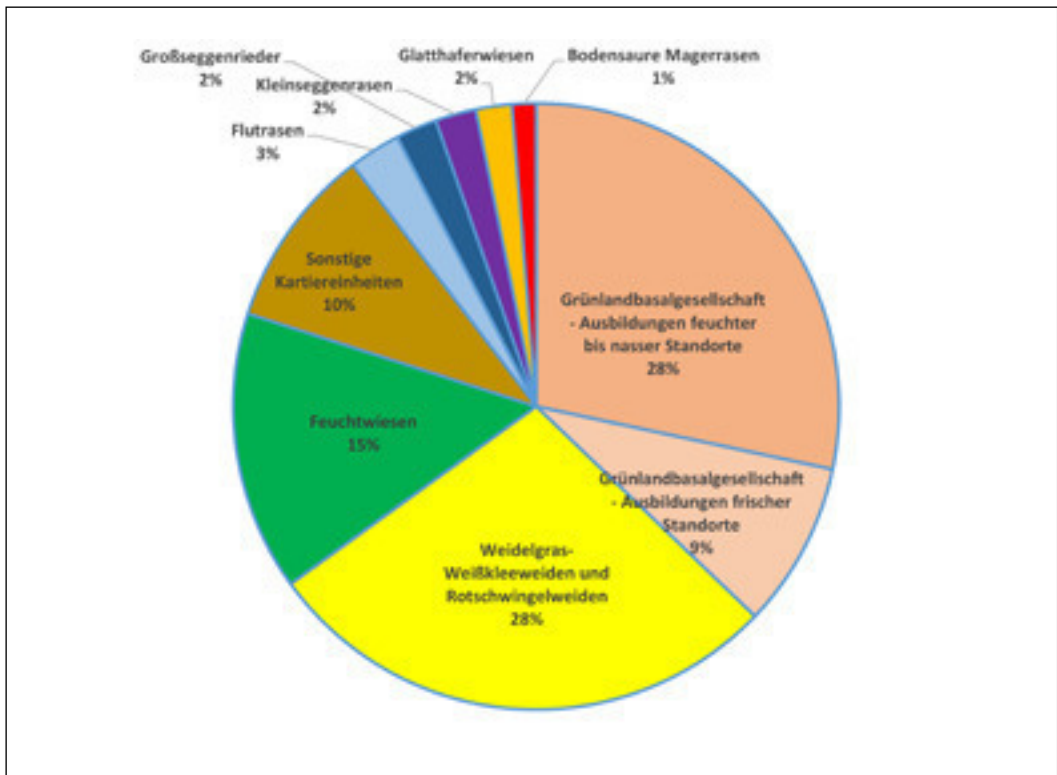
Abb. 17: Anteil der zusammengefassten Grünlandseinheiten im NSG "Großes Torfmoor".
