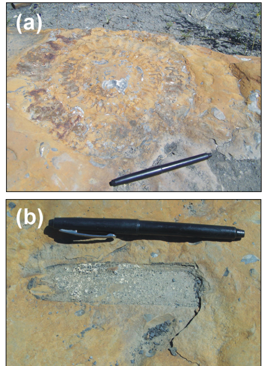
Abb. 7: Fossilien in den Jura-Kalkstein-Blöcken des „Klassenzimmers“. (a): Großammonit Arietites sp., (b): gagatisierter Treibholzrest.
