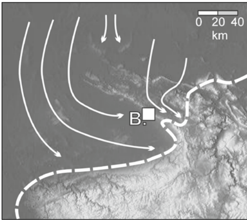
Abb. 4: Eisrandlage während des Drenthe-Stadiums der Saalekaltzeit (245.000 J.v.h.). Die Pfeile zeigen die rekonstruierten Gletscher-Fließrichtungen zwischen Weser-Wiehengebirge und Teutoburger Wald.
