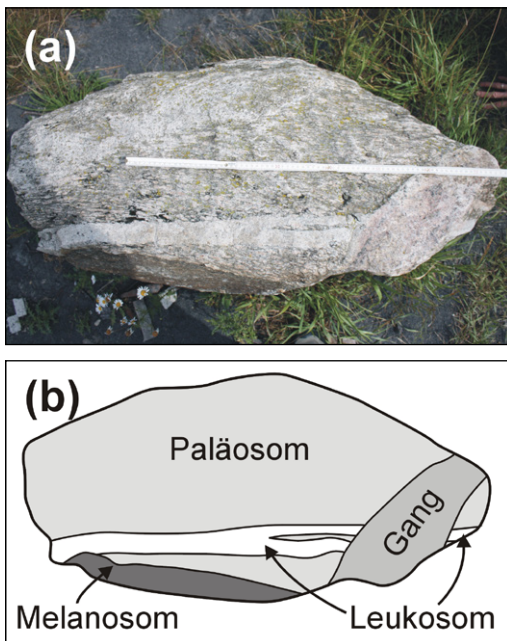
Abb. 6: (a): Migmatit (Stein #48). (b): Skizze der erkennbaren Strukturen. Das Paläosom ist ein stark sigmoidal zerscherter mittelkörniger Gneis. Die migmatitische Textur wird von einem fein- bis mittelkörnigen Gang durchschlagen.
