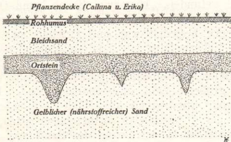
Abb. 2. Ortsteinprofil (schematisch).
