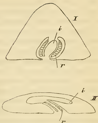
I schematischer Durchschnitt eines, II Pilidium einer Planaria, i Darmkanal, r in I Leibeswand des jungen Nemertes, in II Mundrüssel.
