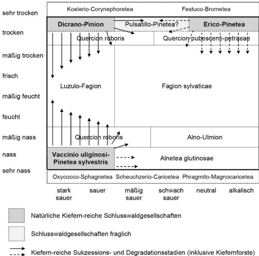
Abb. 1: Ökologische Stellung Kiefern-dominiierter Wälder und Abgrenzung des Dicrano-Pinion in Mitteleuropa. Die durchgezogenen Pfeile charakterisieren die Standorte von Sukzessions- und Degradationsstadien des Dicrano-Pinion. Weitere Erläuterung im Text.
