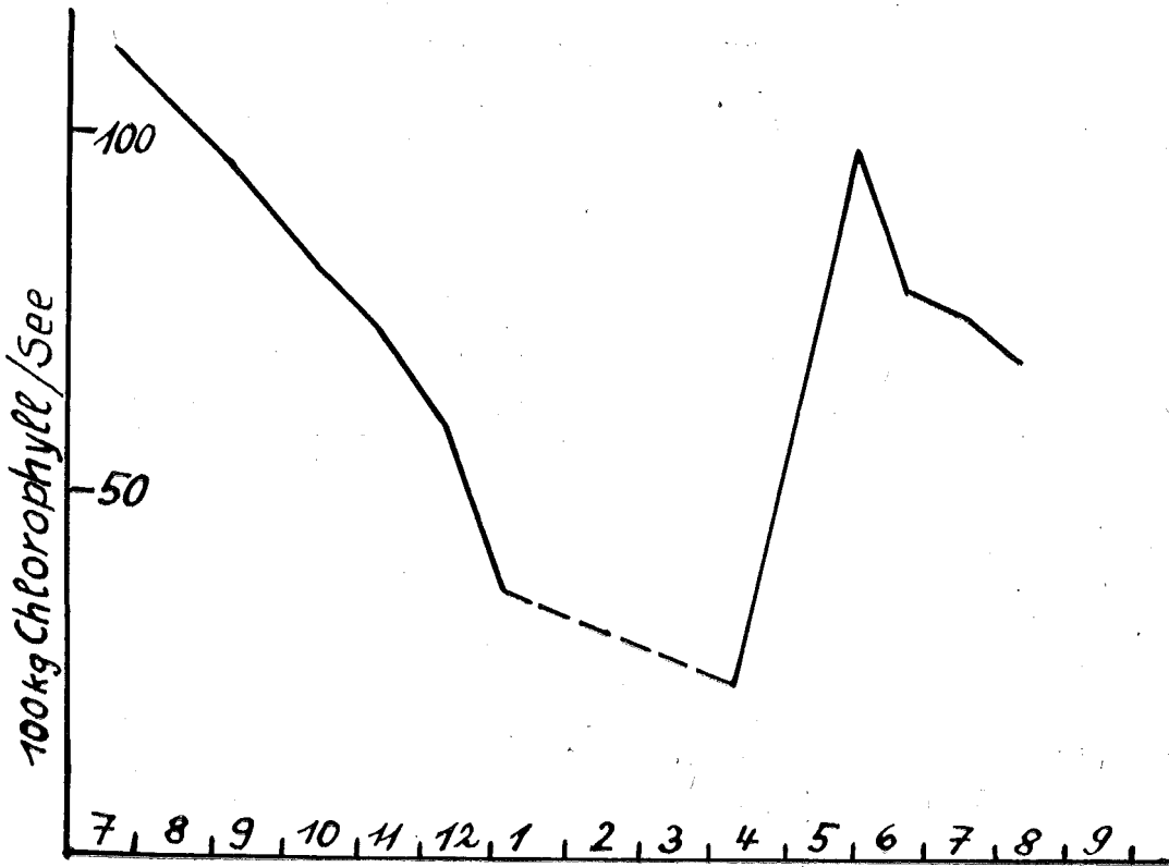
Abb. 3. Jährlicher Gang des Gesamtchlorophylls im Würmsee.
