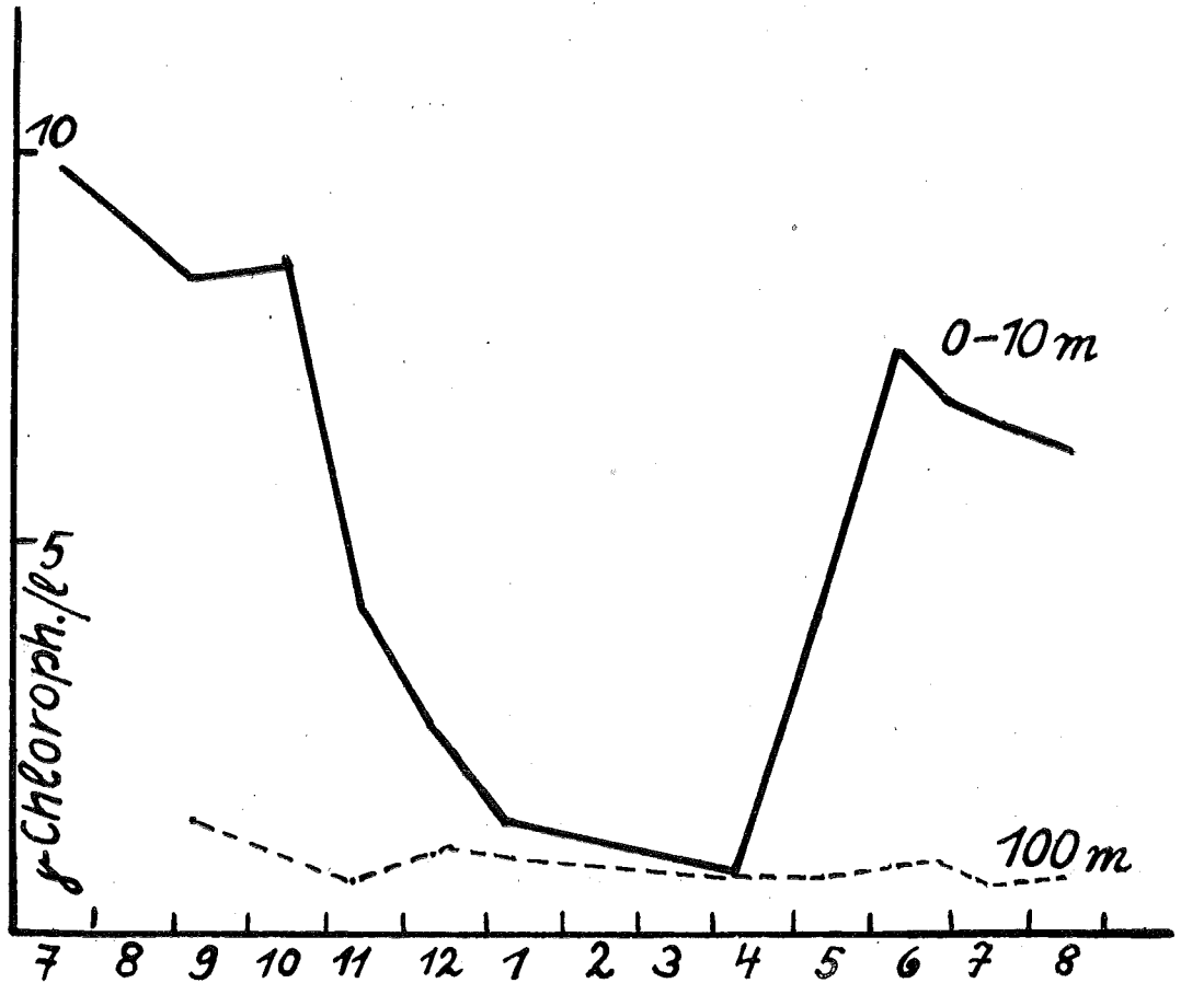
Abb. 2. Jährlicher Gang des Chlorophyllgehaltes im Würmsee an der Oberfläche und in der Tiefe.
