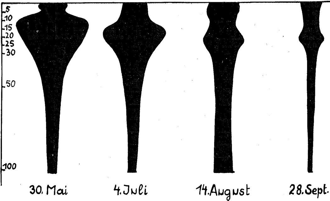
Abb. 4. Vertikale Chlorophyllverteilung im Königssee.
