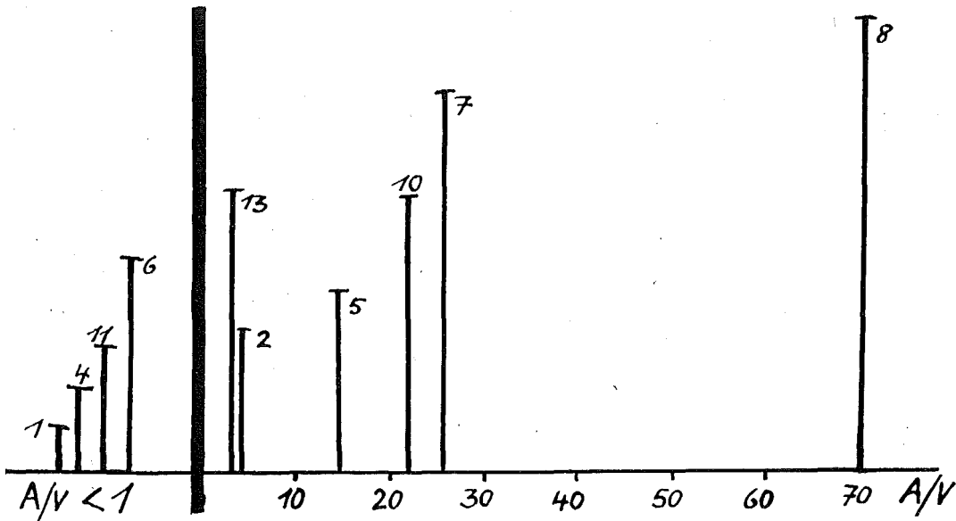
Abb. 6. Beziehung zwischen Besiedlungsdichte und Chlorophyllgehalt in bayerischen Seen. (Nummern der Seen siehe T. I.)
