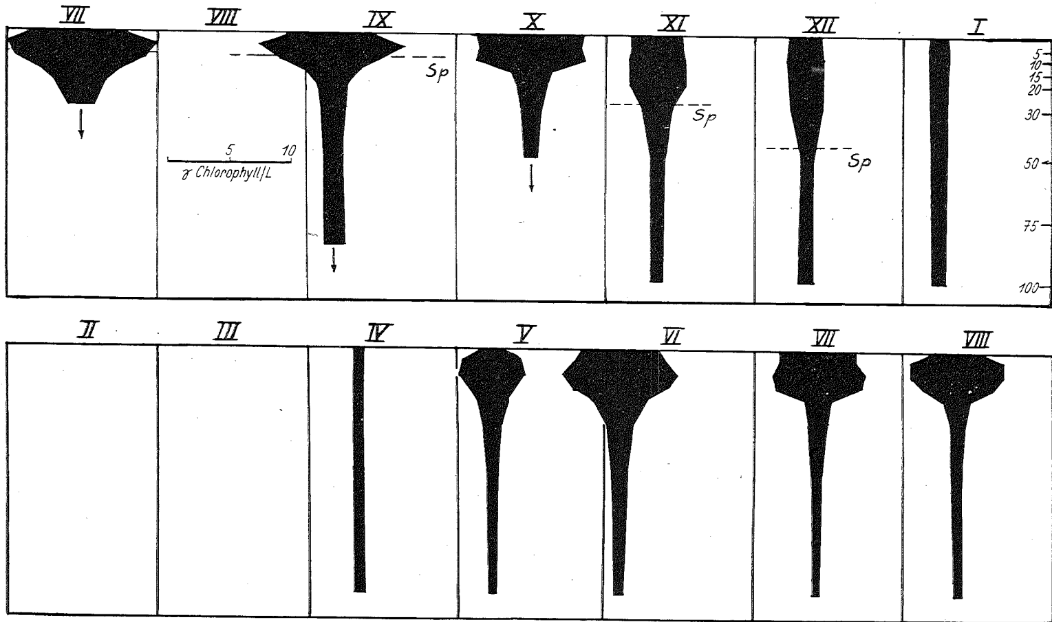
Abb. 1. Vertikale Chlorophyllverteilung im Würmsee (Starnberger See). Sp = Sprungschichte.
