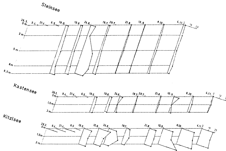
Abb. 8: NITRIT-N-GEHALT Tiefenprofil
