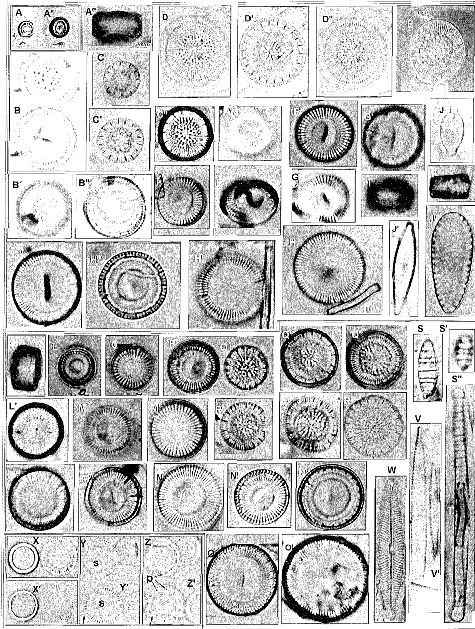
Abb. 3: Kieselalgen aus Bad Tennstedt (A-W) und Cyclotella operculata in Hustedt's Fossil Material (X-Z'). Masstab = 5 µm (exkl. W: 52 µm lang). A-J'' aus dem Kurpark-Teich in Tennstedt [A (Schale mit einem glatten Mittelfeld), A' (Schale mit einem punktierten Mittelfeld), B, C-E ( Cyclotella comta ), A', B', F-I ( C. kützingiana ), h ( Gomphonema sp. 1), h' ( Synedra sp.), I' (Frustule von C. comta ?), J ( Achmanthes exgua ), J' ( Gomphonema sp. 4), J'' ( Stirella sp.)]. K-W aus Graben [K-P ( C. kützingiana ), Q-R'' ( C. comta ), S-S'' (drei Diatoma spp.), T ( Gomphonema sp.1), V-V' (zwei Nitzschia spp.), W ( Navicula sp.)], X-Z' [( Cyclotella operculata in zwei Fokussierungen; s (zentrale Punkte), p (Höcker in Perlenreihe)].
