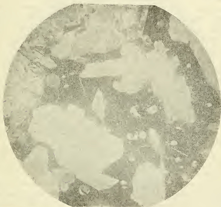
Fig. 5. Gediegen Kupfer in den rundlichen Manderräumen und in der Grundmasse des Diabasporphyrits der Mina Mercedes bei Algodones.
