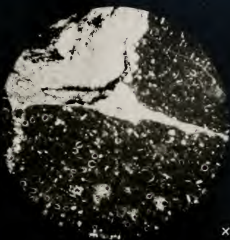
Figur I Calpionella alpina Lorenz
