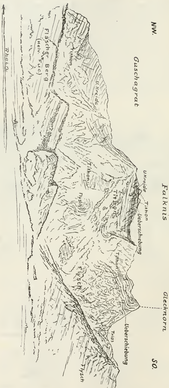
Fig. 12. Ansicht des Falknis von Ragaz aus.
