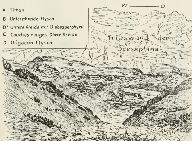
Fig. 15. Geologische Ansicht des östlichen Teils der Quetschzone auf der Alp Fasons.
