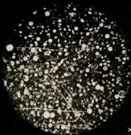
Figur II Pithonella ovalis Kaufm.sp.
