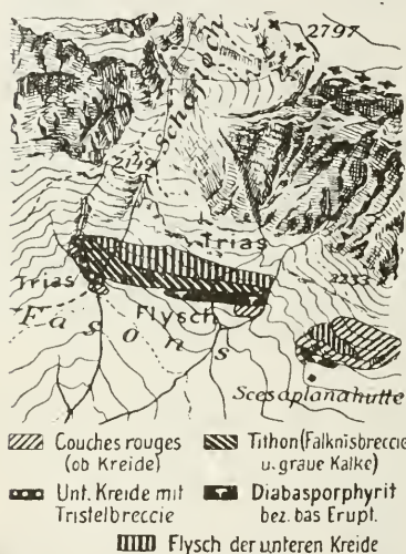
Fig. 13. Geologische Kartenskizze der Alp Fasons. 1:50000.
