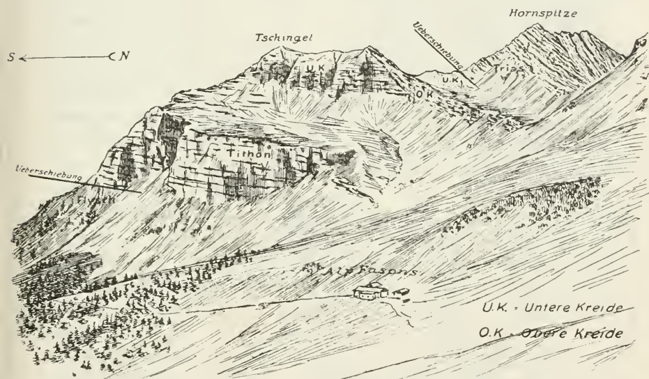
Fig. 11. Ansicht des Tschingel. Ueberschichtung der Trias über Kreide und des Tithon über Flysch.
