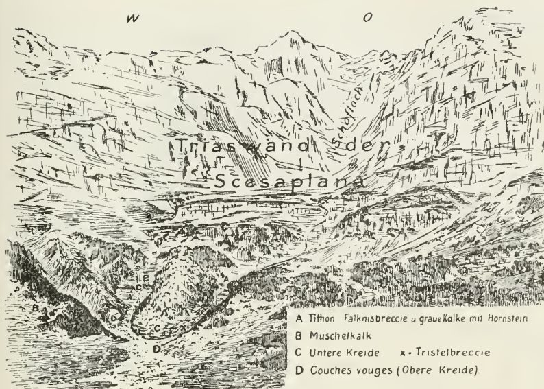
Fig. 14. Geologische Ansicht des westlichen Teils der Quetschzone auf der Alp Fasons.
