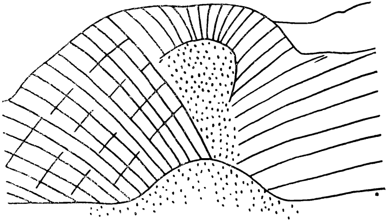
Fig. 2. Schematische Ansicht des durch einen Steinbruch teilweise aufgeschlossenen Hirtsteins.
