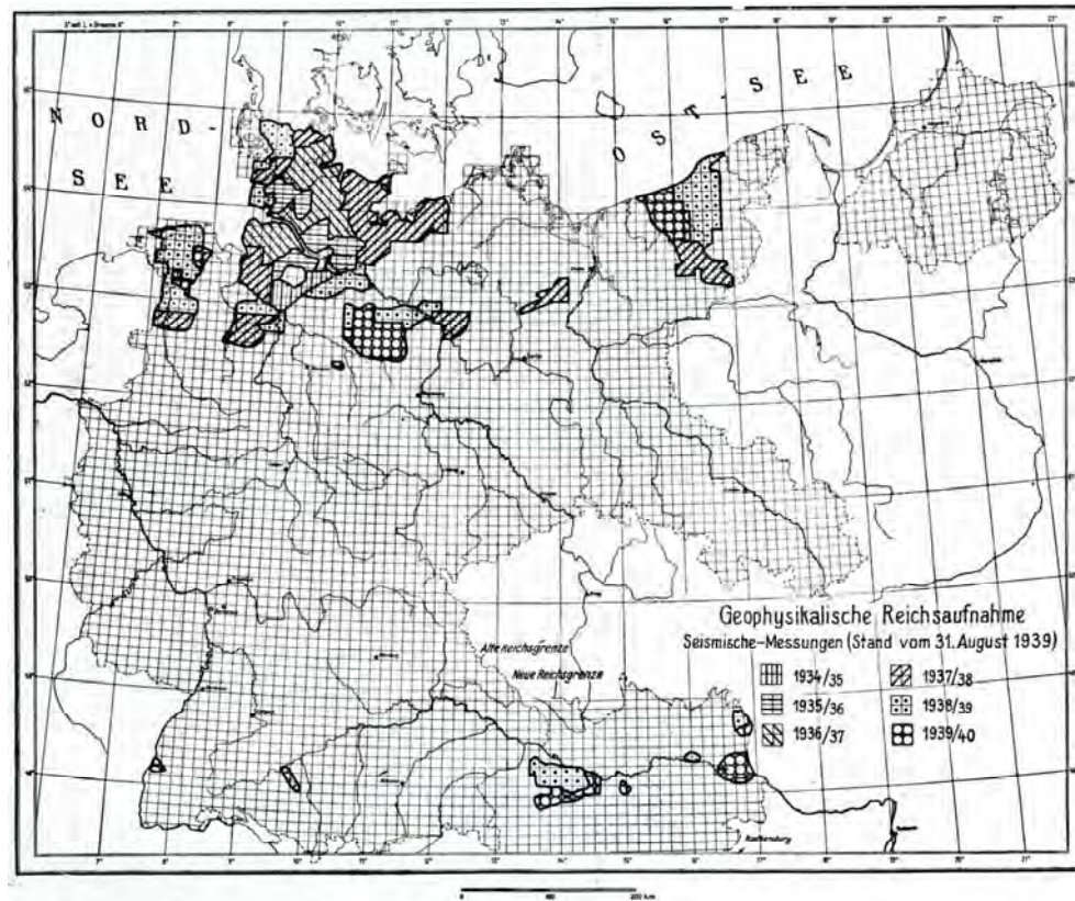
Abb. 56: Geophysikalische Reichsaufnahme: Seismische Messungen (nach BENTZ & CLOSS 1939: 735, Abb. 5)
