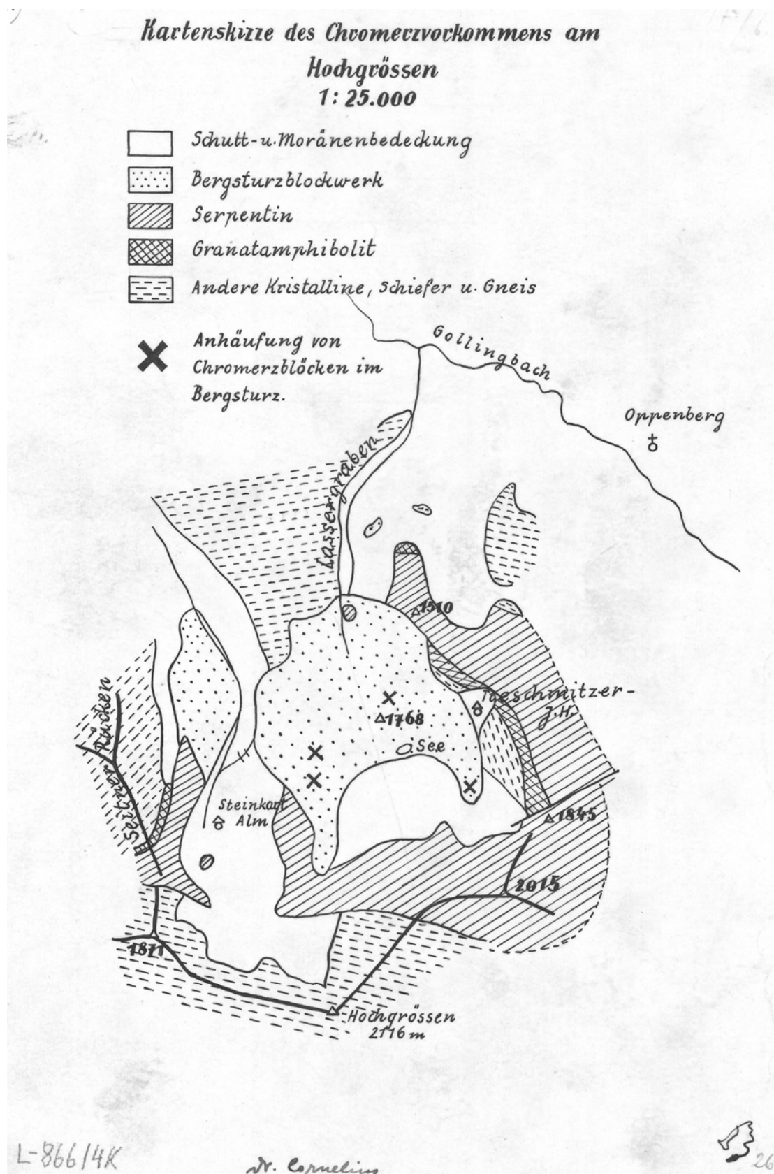
Abb. 22: Kartenskizze des Chromerzorkommens am Hochgrössen (Land Salzburg) von Hans Peter Cornelius (Reproduktion: GBA)
