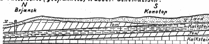
Fig.3 Artesisches (gespanntes) Wasser. Schematisch.
