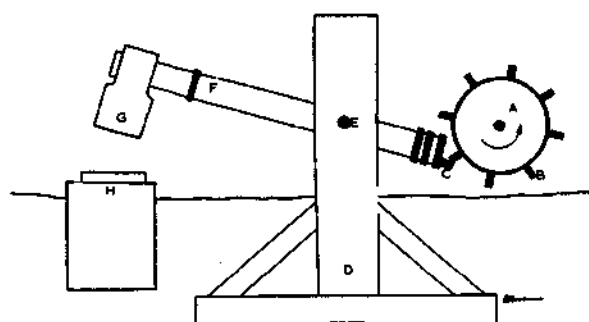
Mechanischer Schwanzhammer
