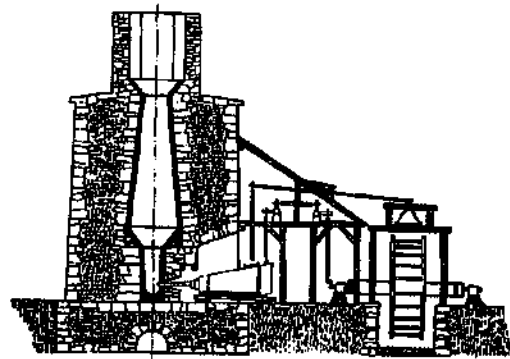
Blasgewölbe im Schnitt
