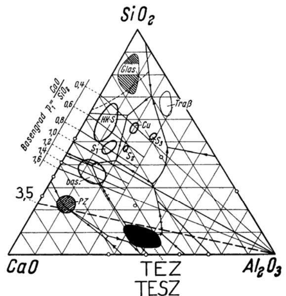
Abb. 5: Dreistoffsystem \text{SiO}_2 - \text{CaO} - \text{Al}_2\text{O}_3 mit Richtwerten für die chemische Zusammensetzung u. a. von Glas, Schlacke des Holzkohlen-Hochofens (HK-S), saure (S1, S2, S3) und basische (bas.) Schlacke des Kokshochofens, Portlandzement (PZ) sowie Tonerde- (TEZ) bzw. Tonerdeschmelzzement (TESZ). Aus KEIL, F. (1949), 35
