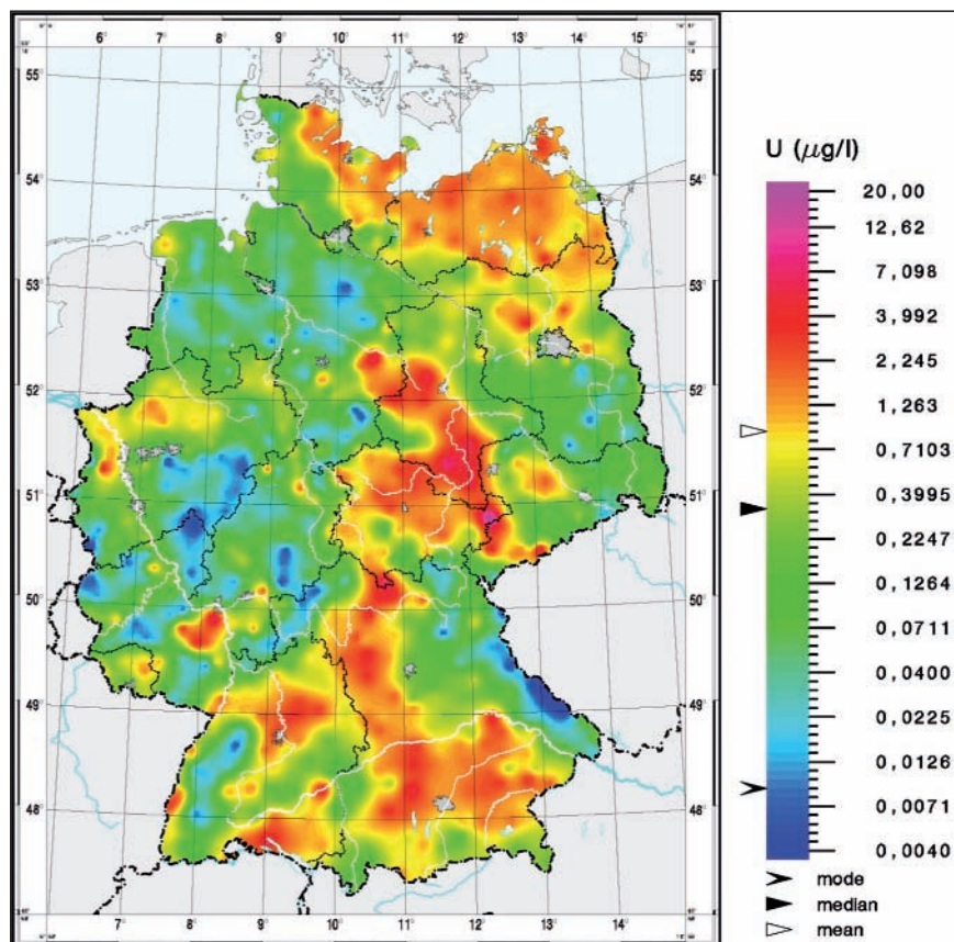
Abb. 1. Uranverteilung in den Oberflächenwässern.
