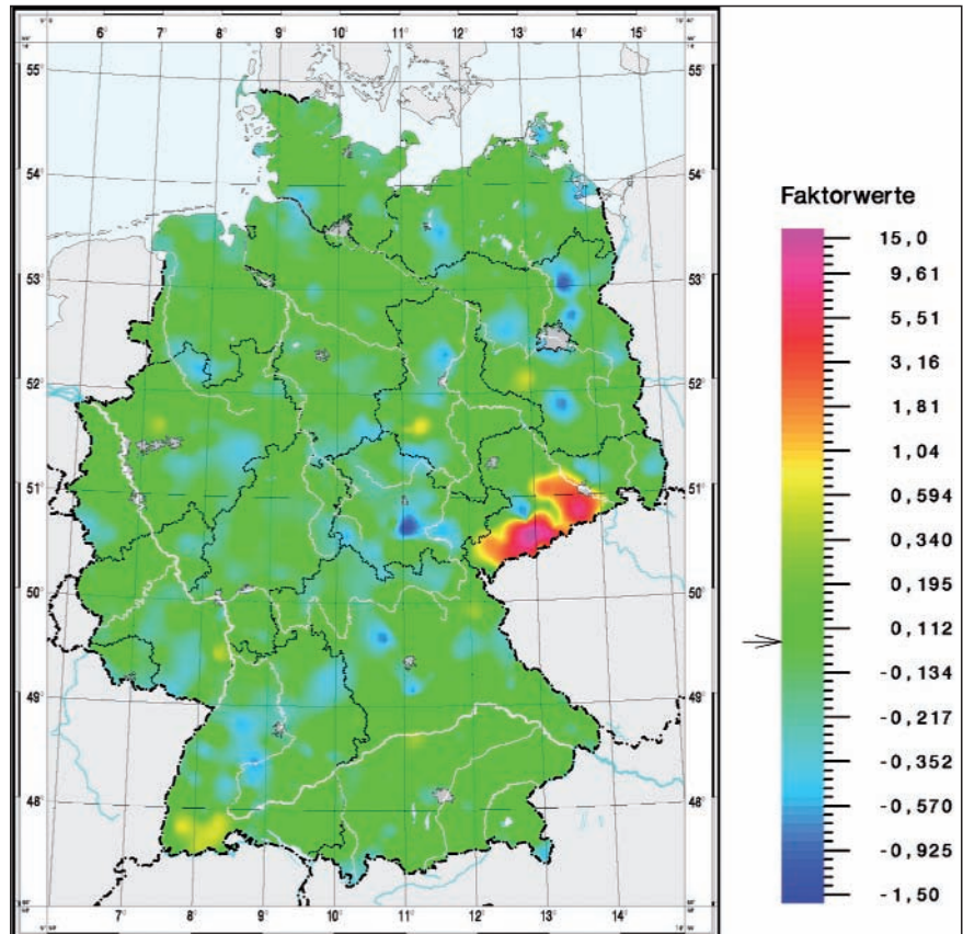
Abb. 2. Faktorwertverteilung des Faktors W-In-As-Sn-Bi-Ta-F in den Bachsedimenten (Mineralisationsfaktor)
