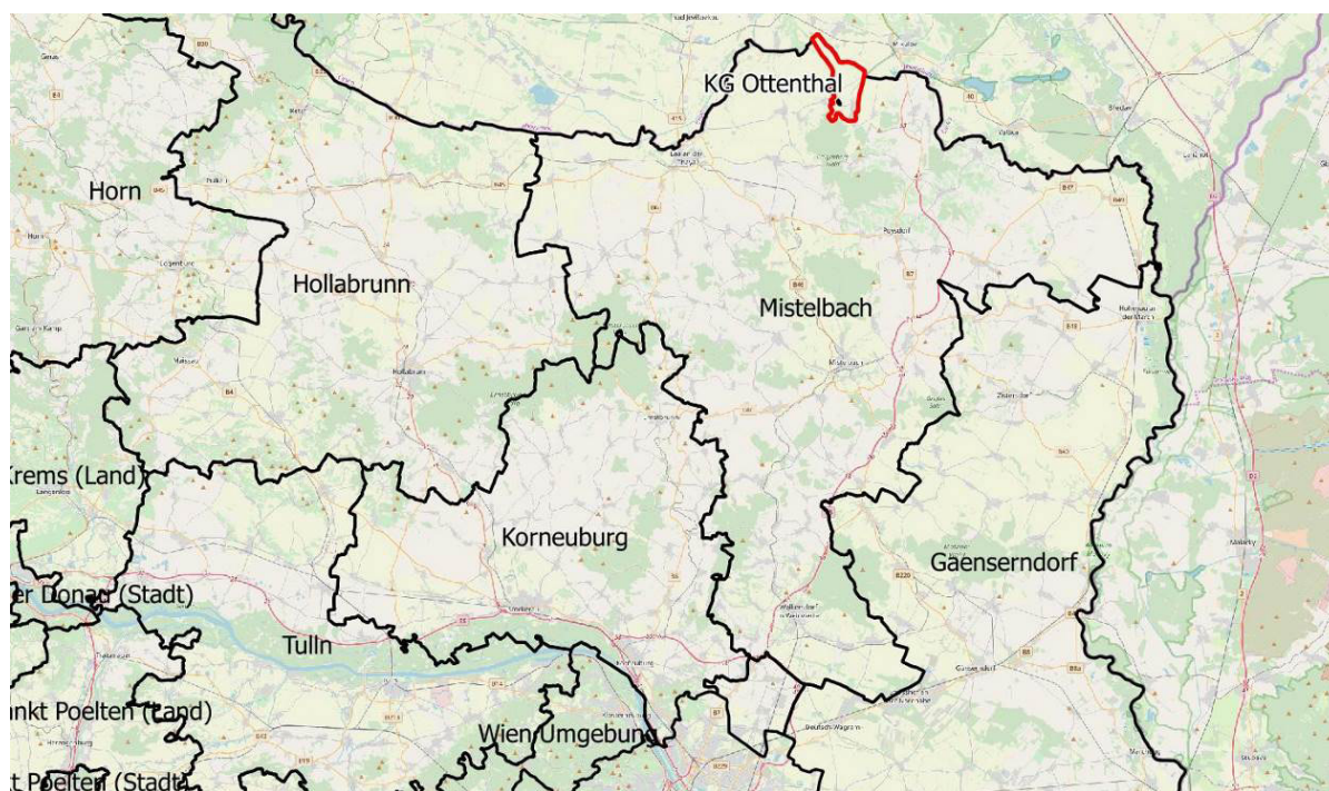
Abb. 1: Lage der Katastralgemeinde (KG) Ottenthal. / Position of the cadastral community Ottenthal. Quelle des Hintergrundbilds: Open Street Map.
