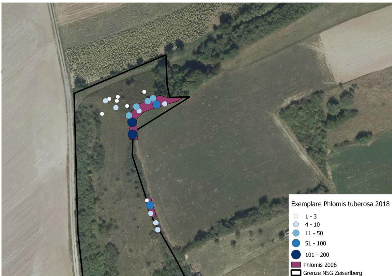
Abb. 3: Lage der Phlomis tuberosa -Bestände 2006 und 2018 sowie Anzahl der blühenden Exemplare 2018. / Location of the Phlomis tuberosa stands in 2006 and 2018, as well as the number of flowering specimens in 2018. Quelle des Hintergrundbilds: Google Earth.
