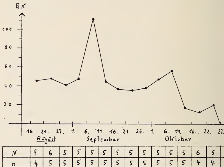
Abb. 3. Verlauf des Limikolenzuges im Herbst 1961, Klärteich Böspërde i. W. (N = Kalendertage, n = Beobachtungstage).
