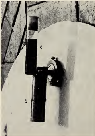
Abb. 2. Aufhängung des Futterröhrens an der Rückseite der Futterscheibe. R = Futterröhren, G = Gegengewicht, das das Röhren bei der Drehung in der senkrechten Lage hält.
