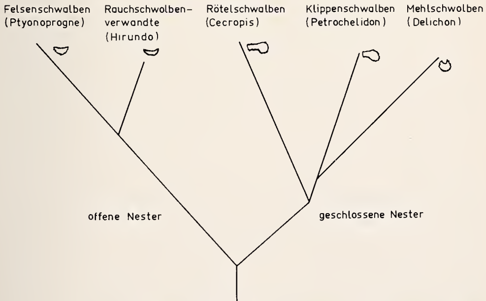
Abb. 2. Vermutliche stammesgeschichtliche Beziehungen der Gattungen der Lehm-nester bauenden Schwalben. Mit schematischer Darstellung der Nestformen.
