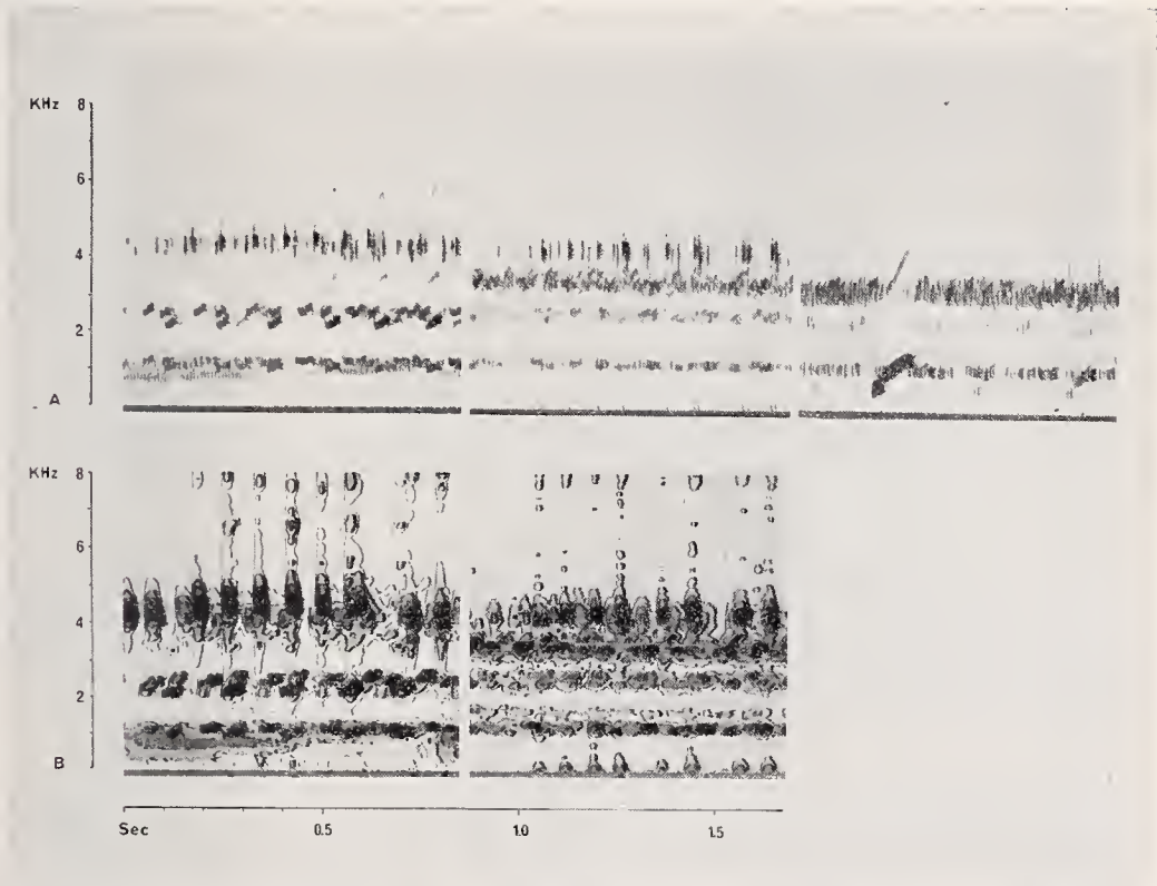
Abb. 3: Klangspektrogramm des Gesamtchors. A li.: Cacosternum boettgeri , Tomopterna marmorata , Bufo garmani , DVP. A Mitte: Cacosternum boettgeri , Tomopterna delalandii , T. marmorata , Okapaue. A re.: T. delalandii , dazwischen Kassina senegalensis , Okapaue. B: „Intensity Contour Display“ des Gesamtchors wie in A (li. und Mitte) dargestellt.
