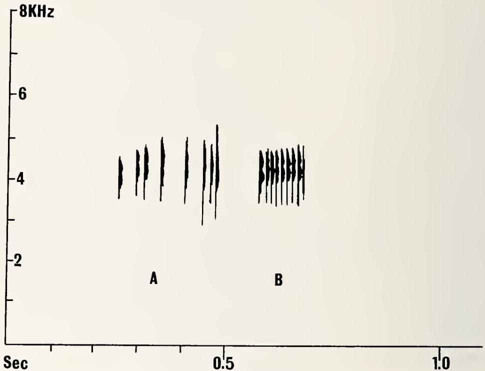
Abb. 2: Klangspektrogramm des Paarungsrufes von Cacosternum boettgeri , Okapae. Ruffolge eines Tieres, Ruftyp A und B.
