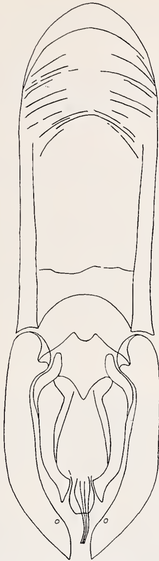
Abb. 1: Saemundssonina minitrans n. sp. Männlicher Kopulationsapparat.
