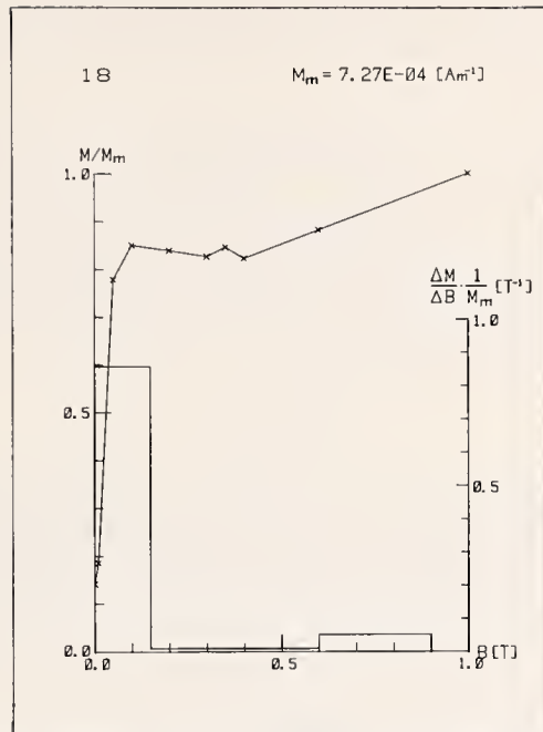
Abb. 3: IRM-Erwerbskurve von Probe 18 ( Clethrionomys ); vgl. Abb. 1.
