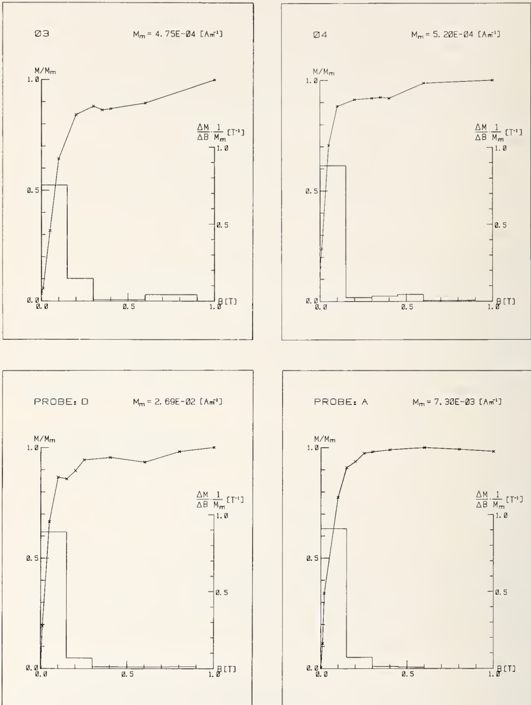
Abb. 1: IRM-Erwerbskurven der Proben von Clethrionomys (Proben 3 und 4), Pitmys (Probe D) und Mus (Probe A). Die Remanenzen (M) auf die maximal erworbene Remanenz (Mm) normiert. Das Histogramm zeigt den Remanenzenerwerb (M) pro Feldstärkerhöhung (B) um jeweils 0.05 T, ebenfalls auf die maximal erworbene Remanenz (Mm) normiert.
