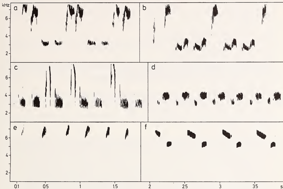
Abb. 3 a–f: Lautäußerungen von Parus fasciiventer (a–e). — a–d) Reviergesang, aufgebaut aus Element-Gruppen, in d) P. major ähnlich (vgl. Abb. 3 f), e) Kontaktrufe während Futter-suche, f) Reviergesang einer Kohlmeise ( Parus major ), (Deutschland). Für f abweichende Skala: oberer Frequenzbereich der hohen Elemente bei 6 kHz. — Vocalizations of Parus fasciiventer (a–e). — a–d) Territorial song, composed of element groups, similar to P. major in d) (see fig. 3 f). e) contact calls while feeding, f) territorial song of Parus major , (Germany). Note different scale in fig. f: upper frequency range of higher elements at 6 kHz.
