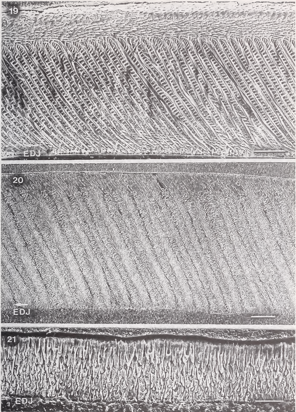
Abb. 21: Procavia capensis , Hyracoidea, rezent. Querschnitt durch das Schmelzband des oberen Inzisiven, das von radialem Schmelz gebildet wird und dem eine dünne prismenlose Außenschicht (PLEX) auflagert (Koe 921, 29368-70; Länge des Balkens 30 \mu\text{m} ).
