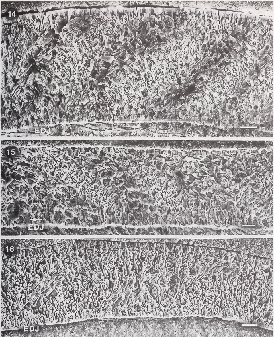
Abb. 14: Palaeolagus sp. Querschnitt durch den I inf. mit durchgehenden HSB. (Koe 668, 28850-52; Länge des Balkens 10 \mu m; EDJ = Schmelz-Dentin-Grenze).
