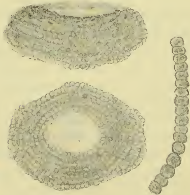
Fig. 4. Anabaena discoidea (Schmidle). Ein Lager von der Seite und von oben gesehen, nebenbei ein Fadenstück mit Heterocyste. — ZEISS, Comp. OC. 2, Apochrom. Obj. 1,25:2,5 ( 200/1 ). Apochrom. Obj. 0,45:4,0 ( 500/1 ).
