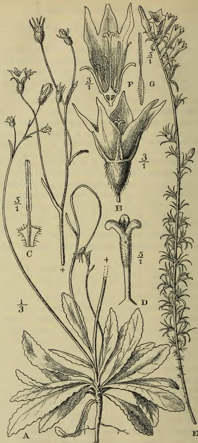
Fig. 3. A—D W. lasiocarpa Schltr. et v. Brehmer. A Habitusbild, B Blüte, C Staubfaden mit verbreiteter Basis, D Griffel mit 6 kleinen Drüsen. — E—G W. fasciculata v. Brehmer. E Habitusbild, F Längsschnitt durch die Blüte mit teilweise abgefallenen Antheren, G Staubfaden mit schwach verbreiteter Basis.
