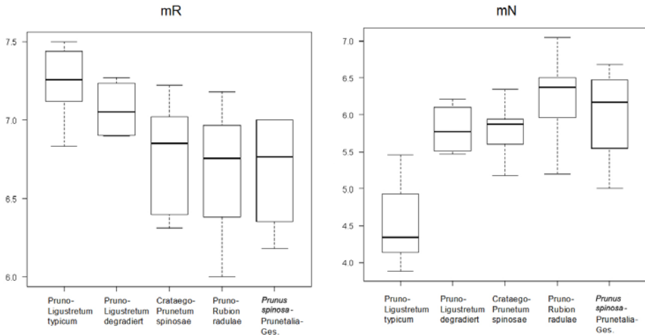
Abbildung 5: Darstellung der mittleren Reaktionszahlen (links) und der mittleren Stickstoffzahlen (rechts) in Tabelle 2 dargestellten Vegetationsaufnahmen als Box-Whisker-Plots. Jeder Plot fasst alle Aufnahmen zusammen, die dem jeweiligen Gesellschaftstyp zugeordnet wurden und zeigt die Spannweite der Werte einer Datenreihe, den Median sowie das untere und obere Quartil.
