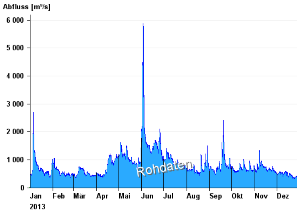
Abb. 2: Abflussgröße am Kraftwerk Braunau-Simbach im Jahr 2013 mit dem Extremhochwasser Anfang Juni (Maximum am 3. Juni 2013 mit 5.875 m³/s)
