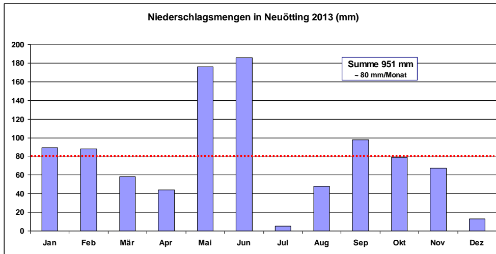
Abb. 1: Monatsverteilung der Niederschläge in Neuötting (eigene Messungen).
