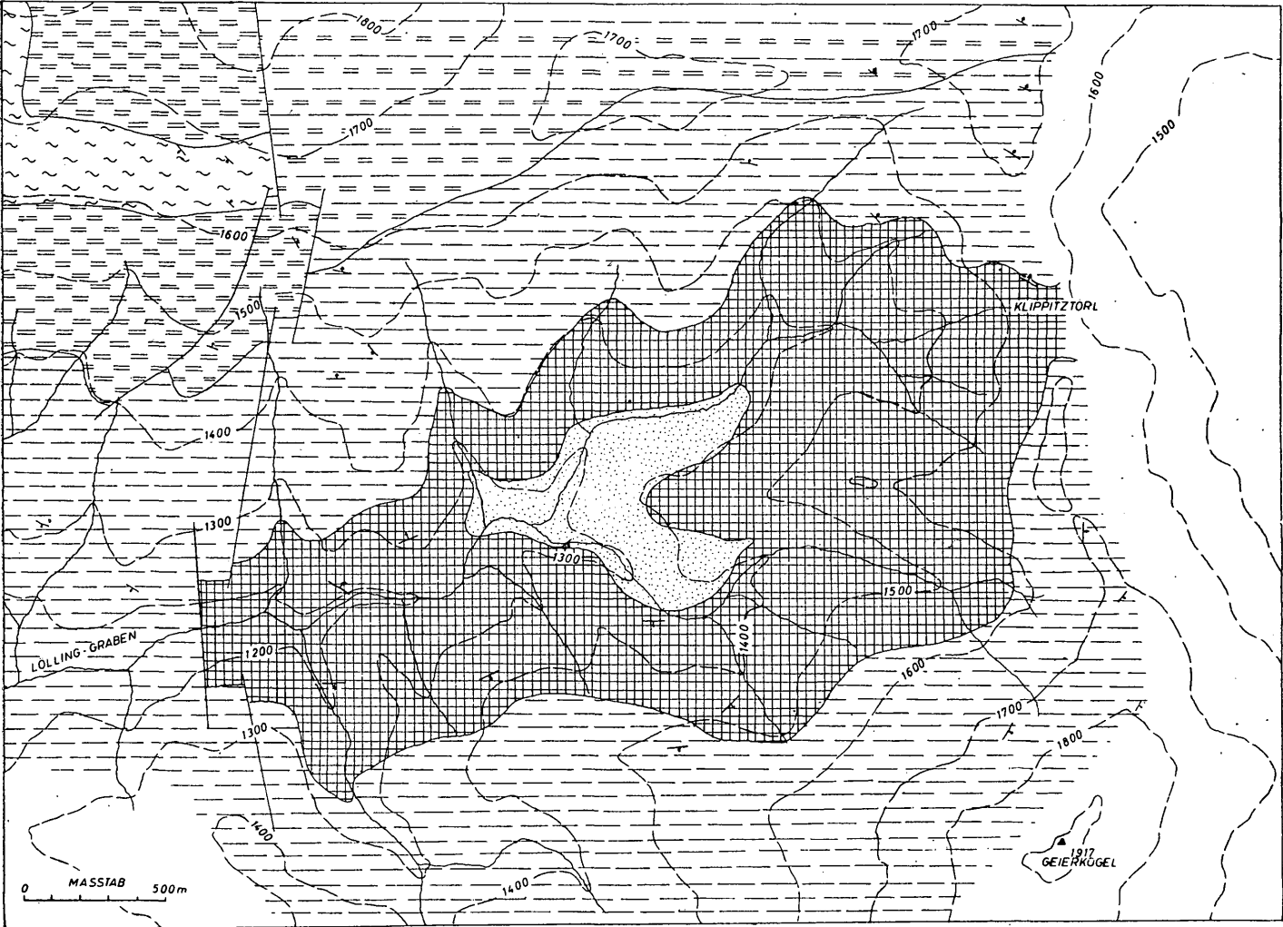
Abb. 2: Das Gewölbe der Stelzing-Marmore im oberen Löllinggraben (Kartierung H. v. KAMP). Punktiert: „Liegendste Serie“; Kreuz schraffiert: Marmorserie der Stelzing; waagrecht gestrichelt: Eklogitserie; doppelt gestrichelt: Disthenflasergneis-Serie; wellig gestrichelt: „Hangendste Serie“; doppelt und einfach gestrichelt: nicht trennbarer Bereich von Disthenflasergneis- und Eklogitserie.
