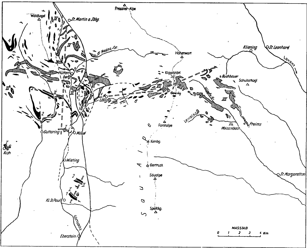
Abb. 1: Bisher bei den Neuaufnahmen kartierte Grüngestein- und Marmorvorkommen im Bereiche der Sausalpe und ihrer westlichen Nachbargebiete. Senkrecht schraffiert: Karbonatgesteine; schwarz: Grüngesteine i. a.; Kreuz schraffiert: Serpentine; durchgezogene oder gestrichelte Linien: Störungen; doppelt gestrichelt: Teilstücke des Idealprofils Abb. 6; die römischen und arabischen Ziffern entsprechen den ebenso nummerierten Komplexen in Abb. 6.
