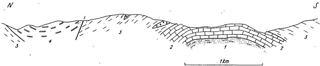
Abb. 3: Profil durch das Gewölbe der Stelzing-Marmore im oberen Löllinggraben (nach H. v. KAMP). — 1 = Liegende Schiefergneise, 2 = Stelzing-Marmore, 3 = Eklogitserie, 4 = Disthenflasergneis.
