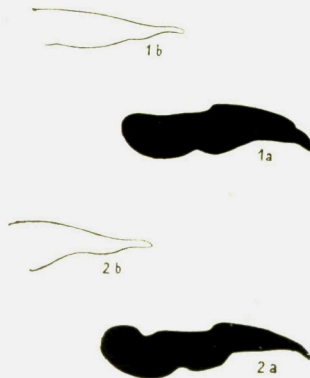
Abb. 1. Choleva vornatscheri Schweig. a) Ventralzahn des Innensackes, Profilansicht, 160 \times . — b) Penisspitze, Profil, 160 \times .
