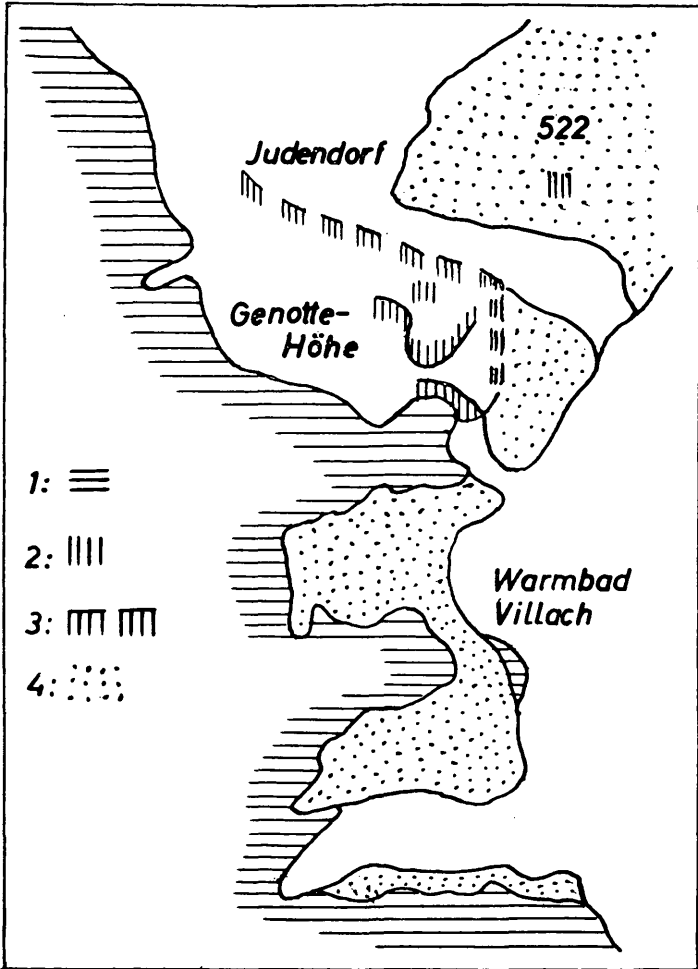
Abb. 1: Geologische Skizze des Gebietes um Warmbad Villach nach J. STINY, 1937: ① Sichtbare Trias der Villacher Alpe — ② Aufgeschlossenes Jungtertiär — ③ Vermutete Umgrenzung des jungtertiären Unterbaues der Genotte- höhe — ④ Verbreitung der Judendorfer Flur (westlich ober den Kur- anstalten von Warmbad Villach die Napoleonwiese, nördlich davon der Jesefeldrain und jenseits des eingeschnittenen Abflusstales die Terrasse der Höhe 522).
