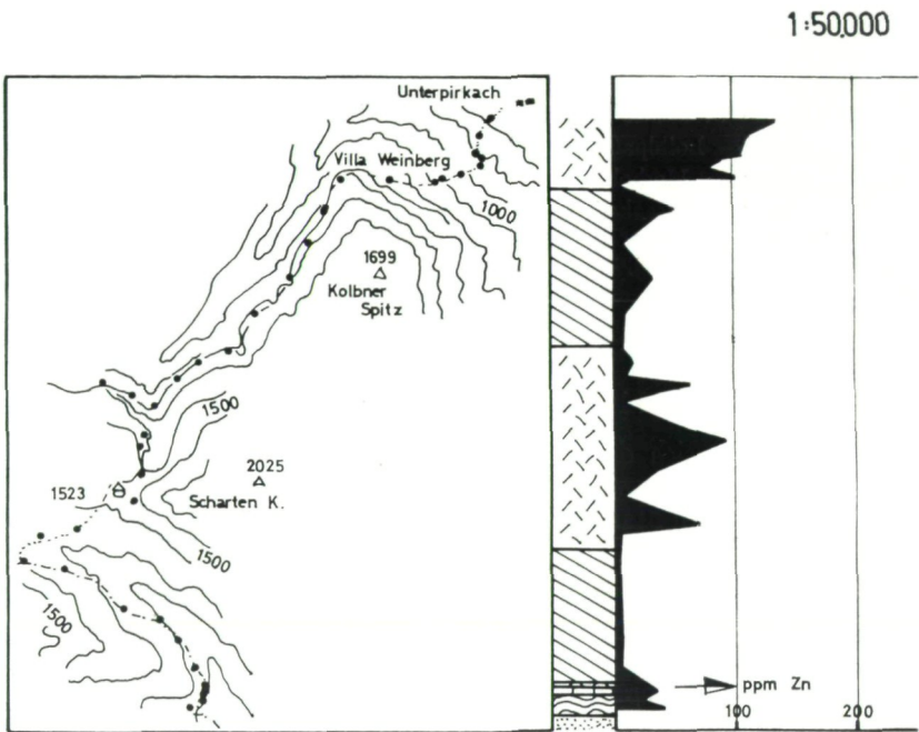
Abb. 1: Profil 4.
