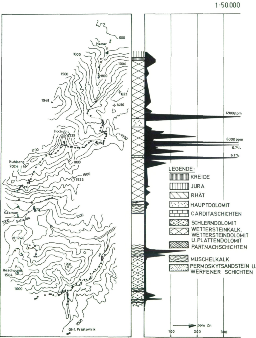
Abb. 4: Profil 16.
