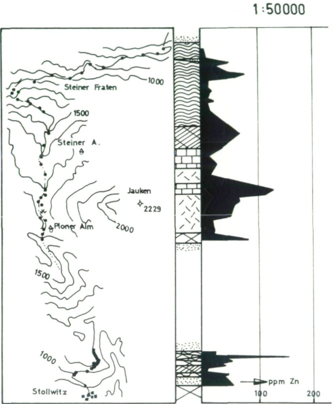
Abb. 2: Profil 6.
