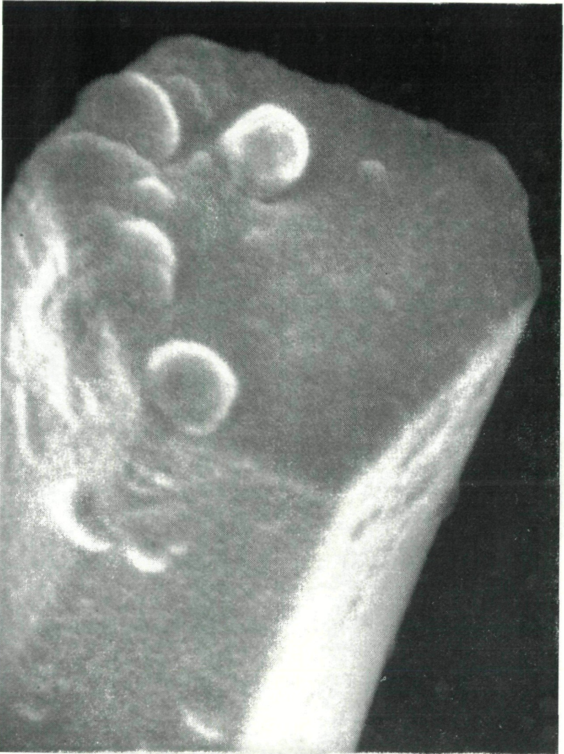
Abb. 7: Stärkste Vergrößerung (etwa 57600 x) eines verbogenen Erionitfadens liefert eindeutig sechsseitig begrenzte Prismen mit glatter Basis. Die kugeligen Warzen sind höchstwahrscheinlich Verunreinigungen von Montmorillonit. Die Dicke des Erionitfadens beträgt etwa 0,0015 nm.
