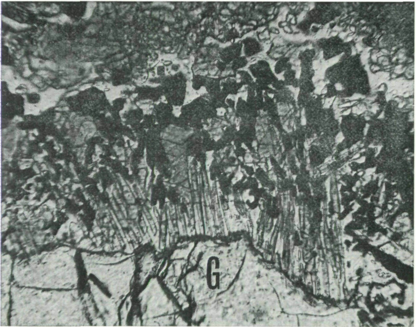
Abb. 3: Eklogitamphibolit mit Hornblendekelyphit. — Geschiebe aus der Drau bei Schloß Hollenburg. — Vergr. = 450 x. Ein Pol., Durchlicht. Vergrößerter Ausschnitt aus Abb. 2, um den Einblick in den Bau der Kelyphitrinde um den Granatporphyroblasten (G) noch anschaulicher zu gestalten.
