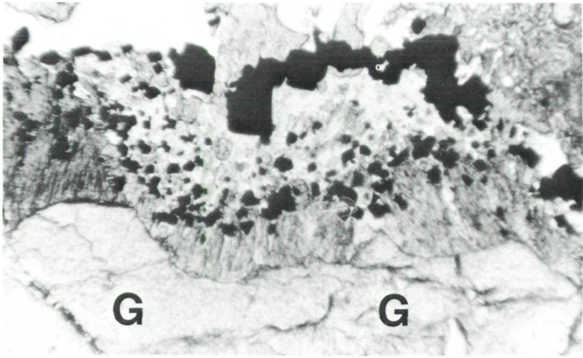
Abb. 4: Eklogit amphibolit, Debanttal, Kärnten. – Vergr. = 140x. Ein Pol., Durchlicht. – Vergrößerter Ausschnitt aus der Kelyphitrinde, siehe Abb. 2, rechts oben. Die Hornblende dieser Rinde um den Granatporphyroblasten (G) ist blauschichtig und an manchen Stellen stengelig-faserig ausgebildet, senkrecht zur Granatoberfläche stehend. Gegen die Kelyphitmitte geht sie in kleinere Körner über, am Kelyphitaußenrand ist die Hornblende gröber körnig. Die Opazitbeteiligung ist relativ hoch. Die Körner treten erst nach einer gewissen Entfernung von der Granatoberfläche auf und werden auch – analog zur Hornblende – nach außen hin gröber. In unserem Detailbild sieht man aber noch eine, wegen der starken Plagioklasbeteiligung, helle Zwischenzone. Manche Opazitkörner zeigen deutlich viereckige Umrisse.
