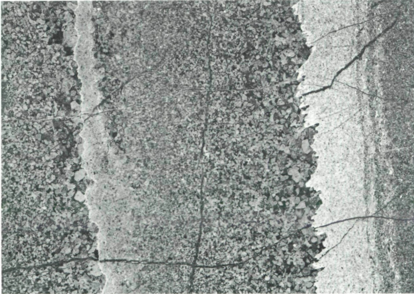
Abb. 3: Gradierter Sedimentzyklus. Die Grenze Grob-Feinanteil ist stylolithisch überprägt. Bankkalkle, Obere Schichtgruppe östlich Eisenkappel. Dünnschliffnegativ, Vergr. 4 X.
