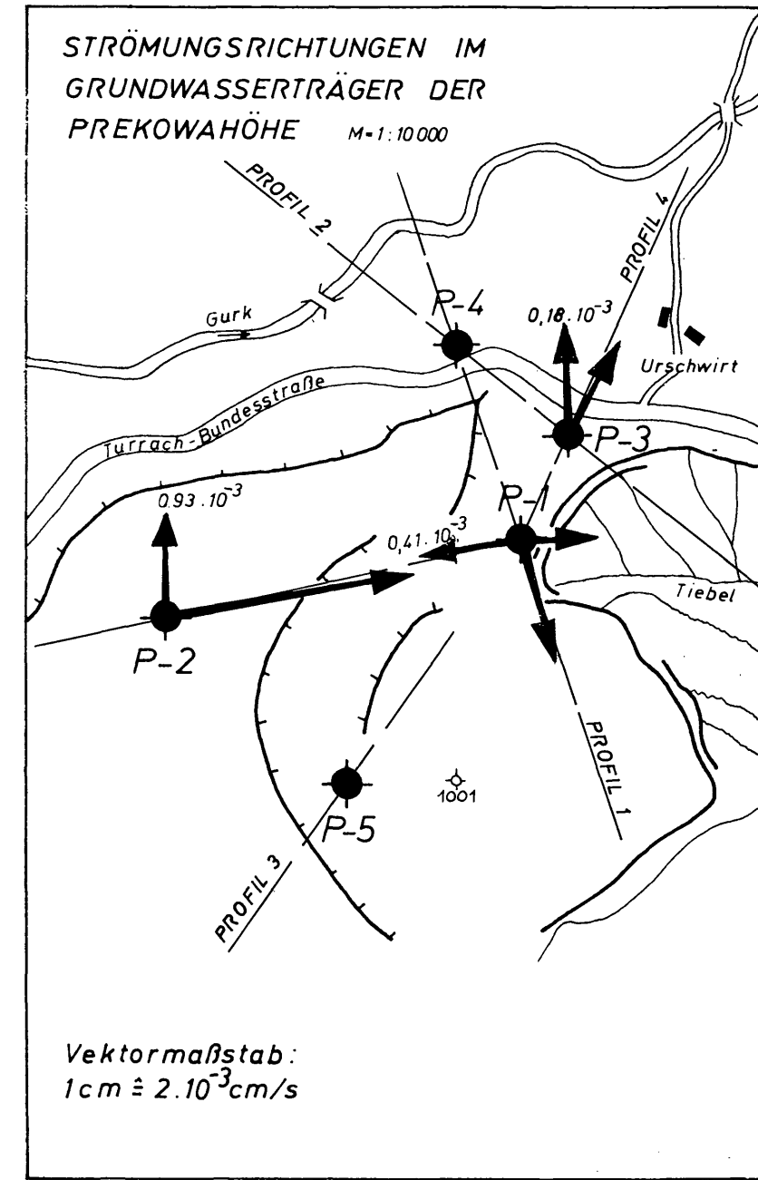
Abb. 2c: Strömungsmessungen
