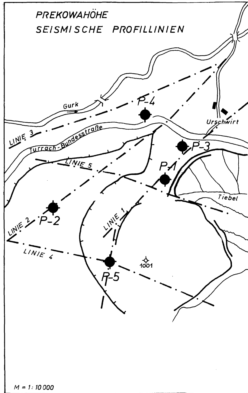
Abb. 2a: Lage der seismischen Profile
