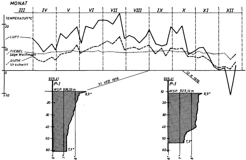
Abb. 4: Luft- und Wassertemperaturen im Bereich der Prekowahöhe (1976).
