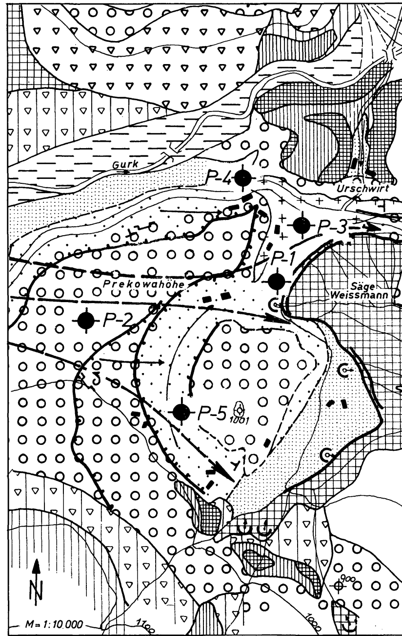
Abb. 2b: Geologische Karte
