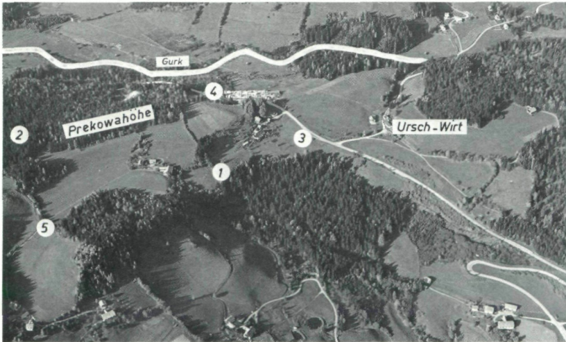
Abb. 1: Prekowahöhe, gesehen vom Süden. 1–5 Aufschlußbohrungen 1976. Südlich der Bohrungen 1 und 3 liegt der auf Kote 890–900 austretende Quellhorizont des Tiebelursprungs. Der Verlauf der Gurk nördlich der Prekowahöhe liegt im Bild oberhalb von Bohrung 4. Foto: Dr. Orel. Freigegeben vom BMFLV mit Zl. 147/9/RAbt.B/76.
