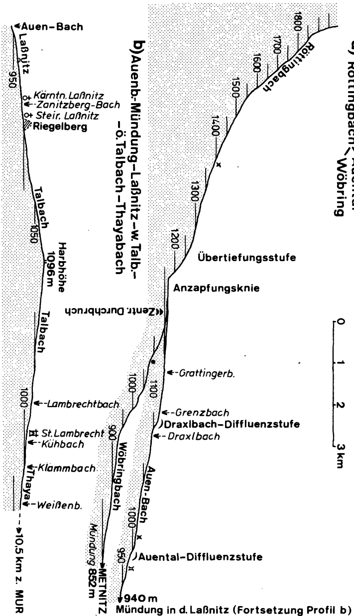
Tafel 1: Tallängsprofile ( der Tallinie entlang, ohne freie Mäander )
