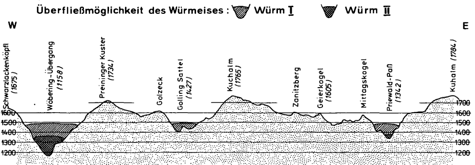
Abb. 2: Die Mur-Metnitz-Wasserscheide vom Wöbring-Übergang bis zur Kuhalm. (Geknicktes Scheitellinien-Profil, 2,5fach überhöht.)
