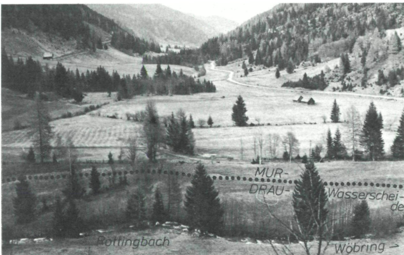
Abb. 5: Blick von der rechten Flanke der Röttingbach-Übertiefungsstufe ins breit ausgestaltete Auental. Im Vordergrund das Knie des zur Wöbering werdenden Röttingbaches. Die Drau-Mur-Wasserscheide befindet sich wenige Meter dahinter.
