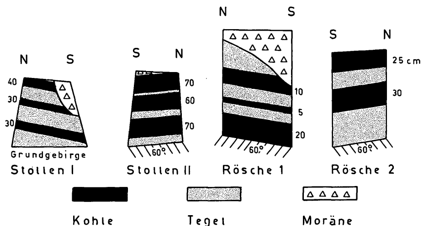
Abb. 2: Sedimentprofile aus der kleinen Podlanig-Terrasse und dem ihr im Westen vorgelagerten kleinen Rücken. Unverändert aus dem Schurfsprotokoll umgezeichnet.
