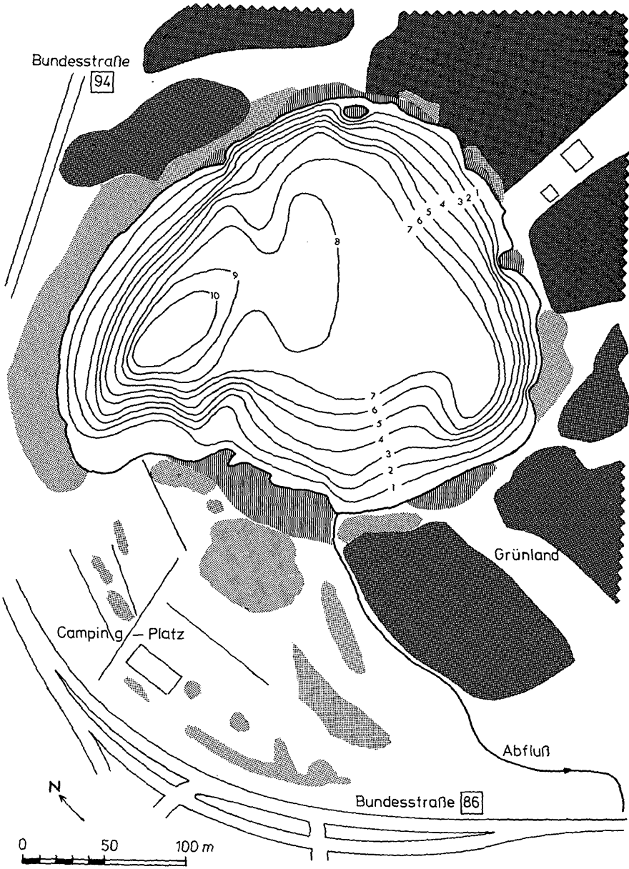
Abb. 5: Tiefenkarte des Vassacher Sees (Legende siehe Abb. 7).
