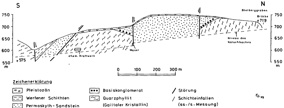
Abb. 2: Geologischer Schnitt durch den Westhang des Nötschbachtals zwischen Bleibergergraben (Höhenpunkt 719) und Höhenpunkt 575.
