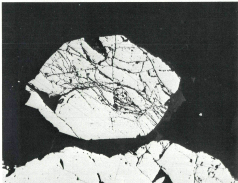
Abb. 3: Zerbrochener Pyritidioblast. Nikolai-Stollen bei Oberdorf. 1 Polarisator, Bildbreite 0,38 mm; weiß: Pyrit, grau: FeOOH, schwarz: Nebengestein.
