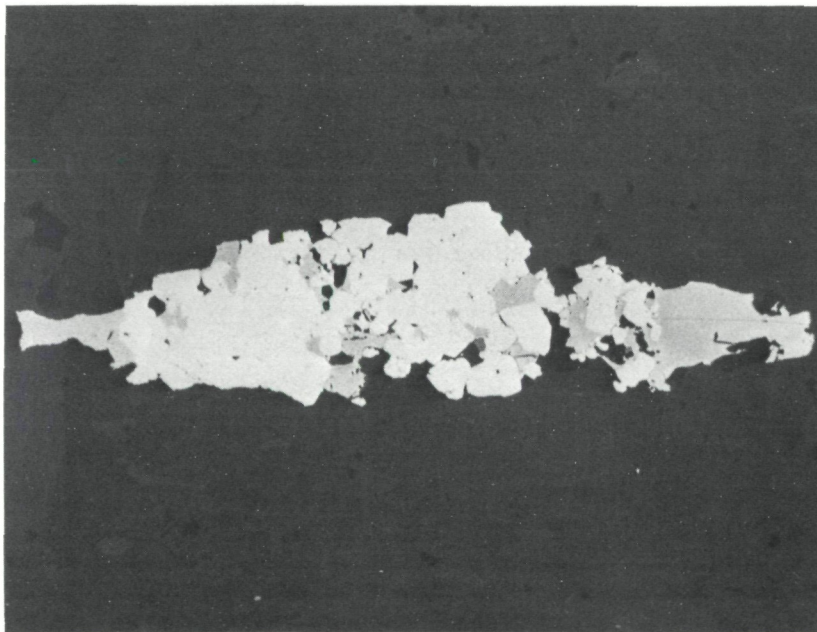
Abb. 6: Schichtparalleles Pyrit-Kupferkies-Aggregat. Klausengrube im Radlgraben. 1 Polarisator, Bildbreite 0,38 mm; weiß: Pyrit, grau: Kupferkies, dunkelgrau: Nebengestein. Foto: S. E. TISCHLER, 1978
