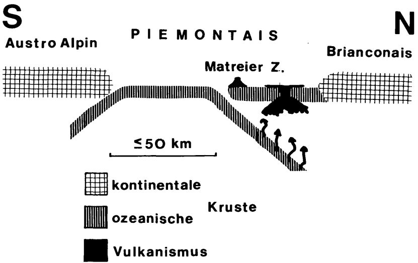
Abb. 15: Schematisches Profil zur Entwicklung der Ablagerungsräume
