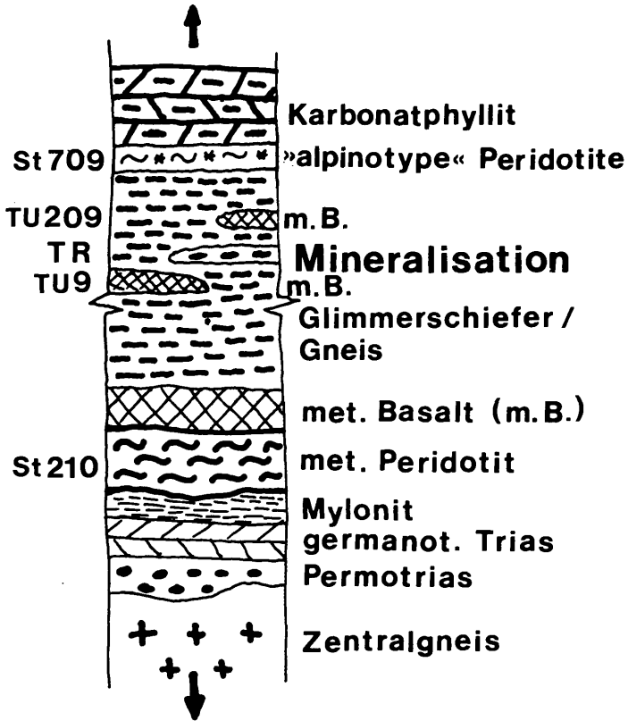
Abb. 14.: Idealisiertes lithologisch–tektonisches Profil durch den Tauernostrand.
