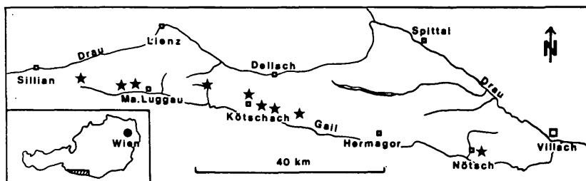
Abb. 1: Lage des Untersuchungsgebietes. Mit * sind jene Profile bezeichnet, in welchen bisher Magnesit in untertriadischen Gesteinen festgestellt werden konnte.
