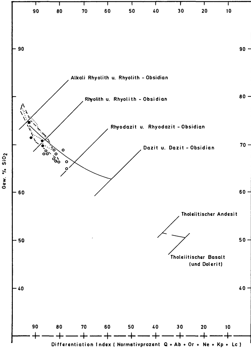
Abb. 6: Die Augengneisproben aus dem östlichen Kristallin des Gailtales im Diagramm SiO 2 -Differentiations-Index nach THORNTON & TUTTLE (1960). Zum Vergleich sind ... (siehe Abb. 2). Die Mittelwerte für Dazit ... (siehe Abb. 5). Signaturen wie in Abb. 2.
