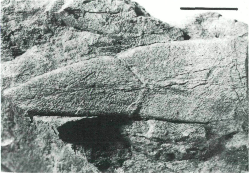
Abb. 8: Neuropteris scheuchzeri HOFFMANN, 1823–1829. Fragment einer Blattspitze.
