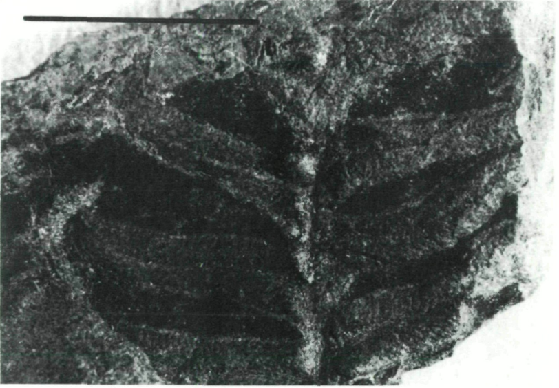
Abb. 13: Alethopteris ambigua LESQUEREUX, 1880.
