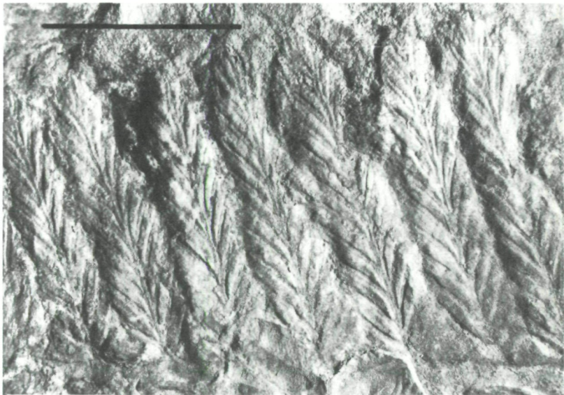
Abb. 4: Pecopteris feminaeformis Auct.
