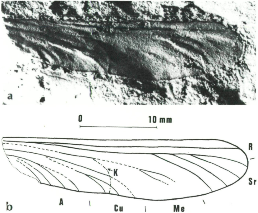
Abb. 1: Arltia carnica n. sp., Holotypus. – Stephanium; Fundpunkt Nähe Kronalpe, Karnische Alpen, Kärnten, Österreich. – a) Photographische Wiedergabe des Flügel-Abdruckes. – b) Rekonstruktion des Flügels. A = Analfeld, Cu = Cubitus, K = postmortal entstandene Knitterfalte, Me = Medialis, R = Radius, Sr = Sector radii.
