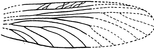
Abb. 3: Arltia eurycubitalis GUTHÖRL, 1940; x 2.0. – Westfal D des Saar-Gebietes (nach GUTHÖRL 1940: Abb. 4; Maschen-Aderung nicht dargestellt). – Die Art ähnelt Arltia carnica unter allen Arltia -Arten am ehesten im Umriß und in der Größe; sie weicht jedoch ab in der Vergabelung der Adern und im kleineren Analfeld.
