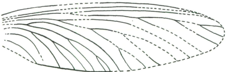
Abb. 2: Arltia obsoleta (GOLDENBERG, 1877); x 1.9. – Westfal C des Saar-Gebietes (nach GUTHÖRL 1934; Abb. 30). – Die Art ähnelt Arltia carnica in der Vergabelung des Sector radii und der Größe des Analfeldes, weicht jedoch ab durch beträchtlichere Flügel-Größe und den dreifach gegabelten Cubitus posterior.
