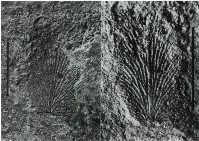
Abb. 33: Linopteris sp.
