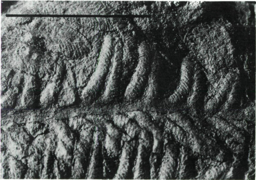
Abb. 28: Alethopteris sp.
