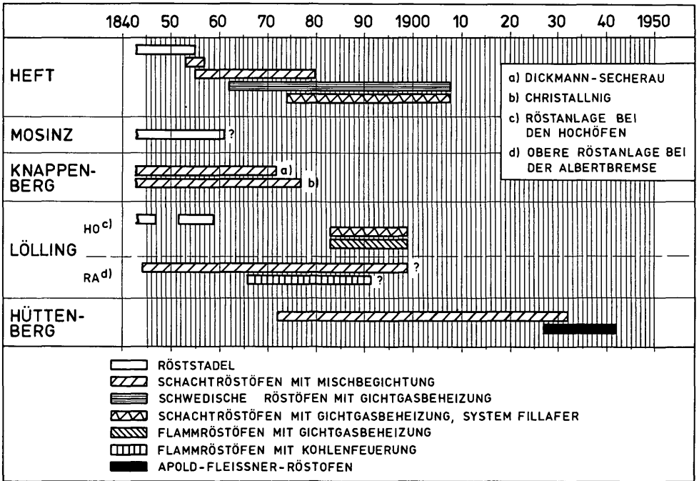
Abb. 22: Die Röstanlagen beim Hüttenberger Erzberg und ihre Betriebsdauer.
