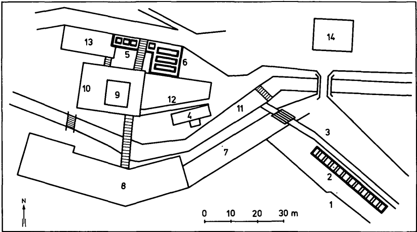
Abb. 2: Lageplan des Eisenwerkes Heft. Vereinfachter Ausschnitt aus einem vom k.k. Bezirksamt Althofen am 30. April 1857 bestätigten Plan (Plan Nr. 593 im Bergbaumuseum Hüttenberg in Knappenberg).
