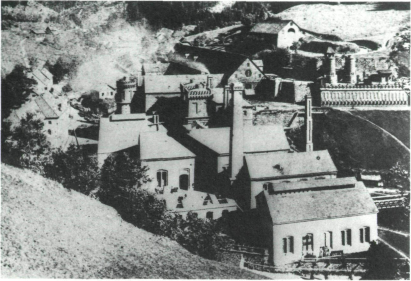
Abb. 5: Eisenwerk Heft um 1890. Ausschnitt aus einer undatierten Fotografie im Bergbaumuseum Hüttenberg in Knappenberg (vgl. Abb. 4). Hintergrund: oben Erzbunker, darunter Kohlbarren, rechts zwei Schwedische Röstöfen und Fillafer'sche Röstanlage mit 24 Öfen. Bildmitte und links: drei Hochöfen und Bessemerstahlwerk. Vordergrund: Gebläse- und Kesselhaus.
